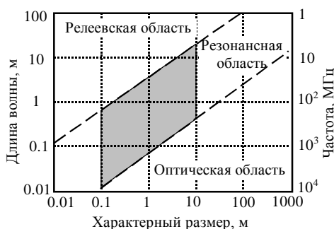
Рис. 1. Взаимосвязь трех областей рассеяния радиолокационных объектов
