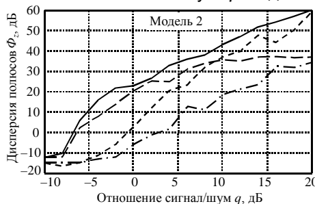
Рис. 5. Зависимость дисперсии полюсов от отношения сигнал/шум. «- - -» – исходный сигнал; «- - -» – АКФ; «- - -» – кумулянты третьего порядка; «—» – кумулянты четвертого порядка
