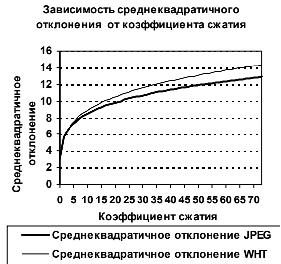
Рис. 2. График зависимостей среднеквадратичного отклонения от коэффициента сжатия для разработанного алгоритма и стандартного алгоритма JPEG
