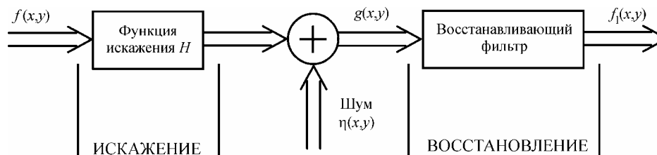
Рис. 1. Модель процесса искажения / восстановления изображений
