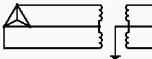
Рисунок Б.1 — Схема включения однофазных неземляемых двухобмоточных трансформаторов в трехфазных электрических сетях с изолированной нейтралью и напряжением 3 — 35 кВ
